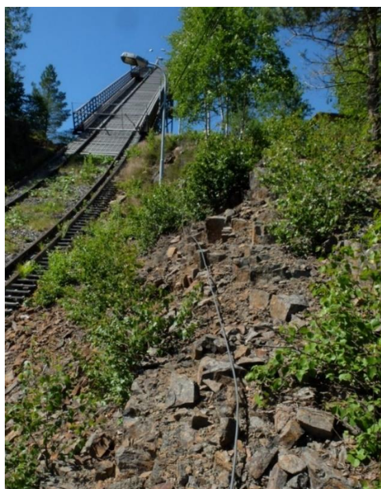
Tilførselsledning til fartsstillaset falt ned.
