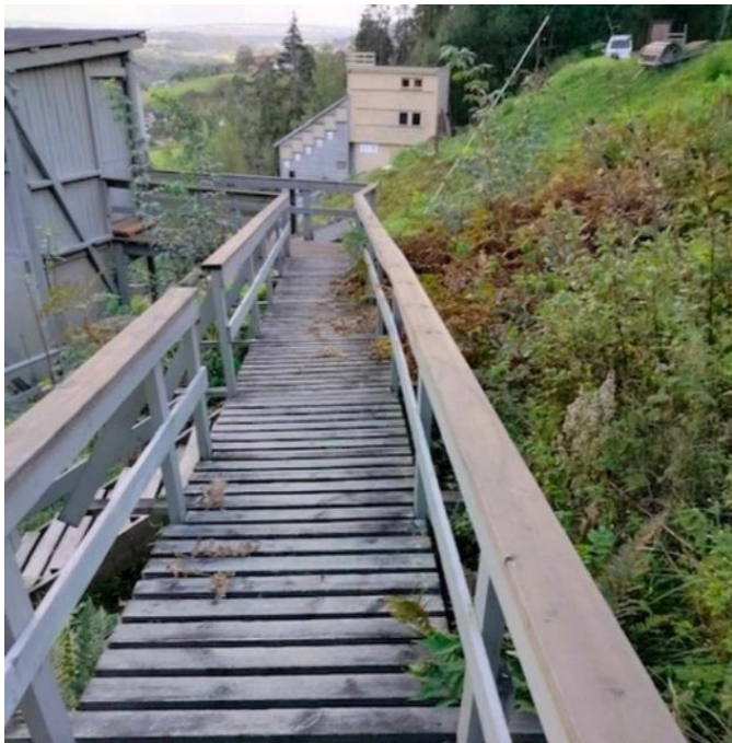
Håndrekke på gangveien til kongtribunen skiftet ut., Foto Cany Bygg
