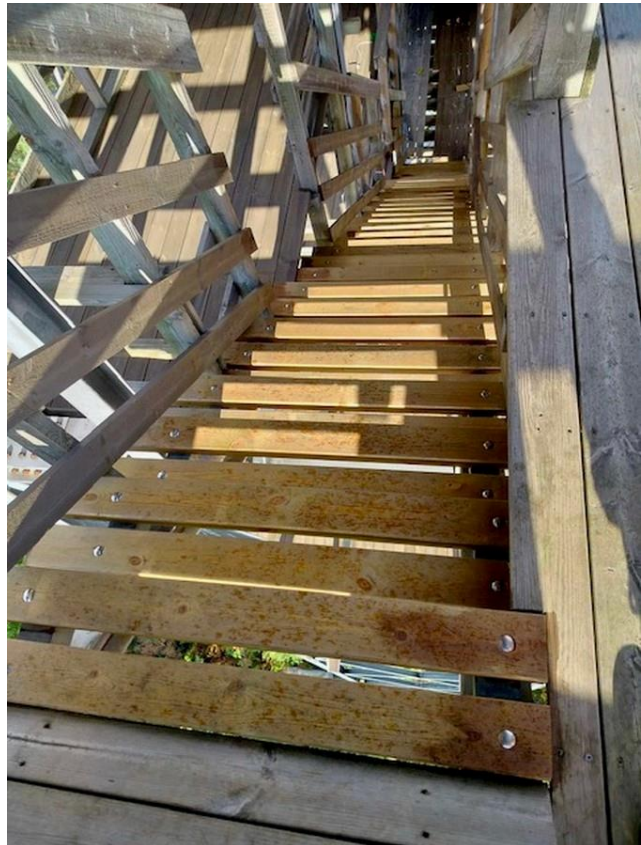
Nest øvre indre trapp fra avsats 1 forbi avsats 2, 3 og 4 til avsats 5. Tv. sett oppover, th. nedover.
